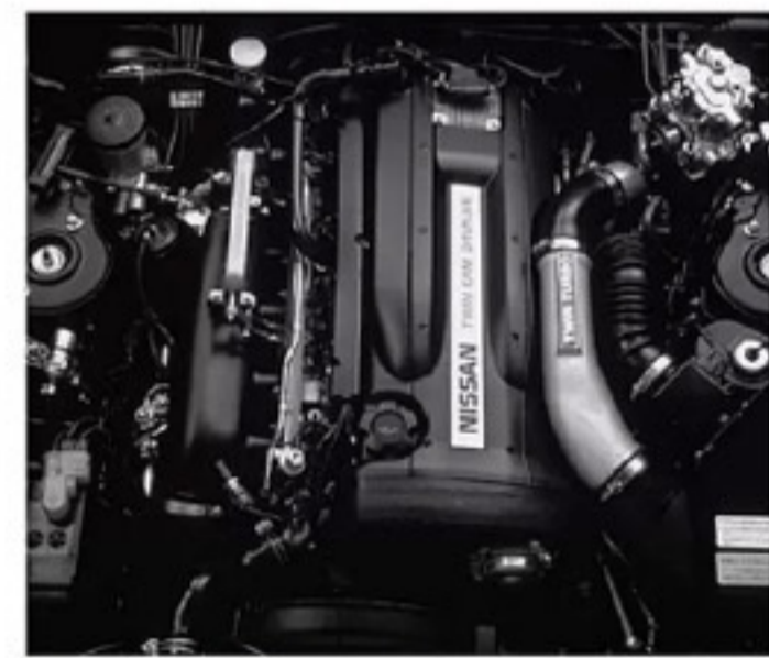
RB26DETT型ツインターボエンジンが採用された。最高出力は当時の自主規制上限となる280馬力！
